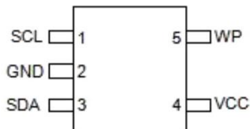
SOT-23-5
