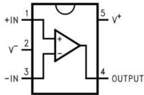
SOT-23-5
